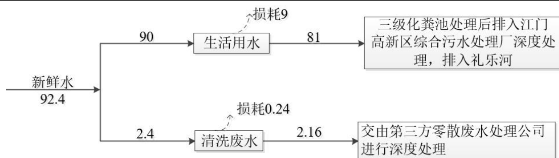
7、VOCs 平衡图（单位：t/a）
