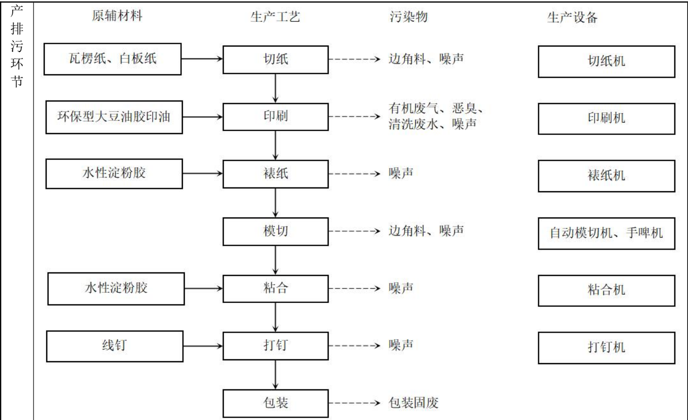
图2-2 生产工艺流程图
