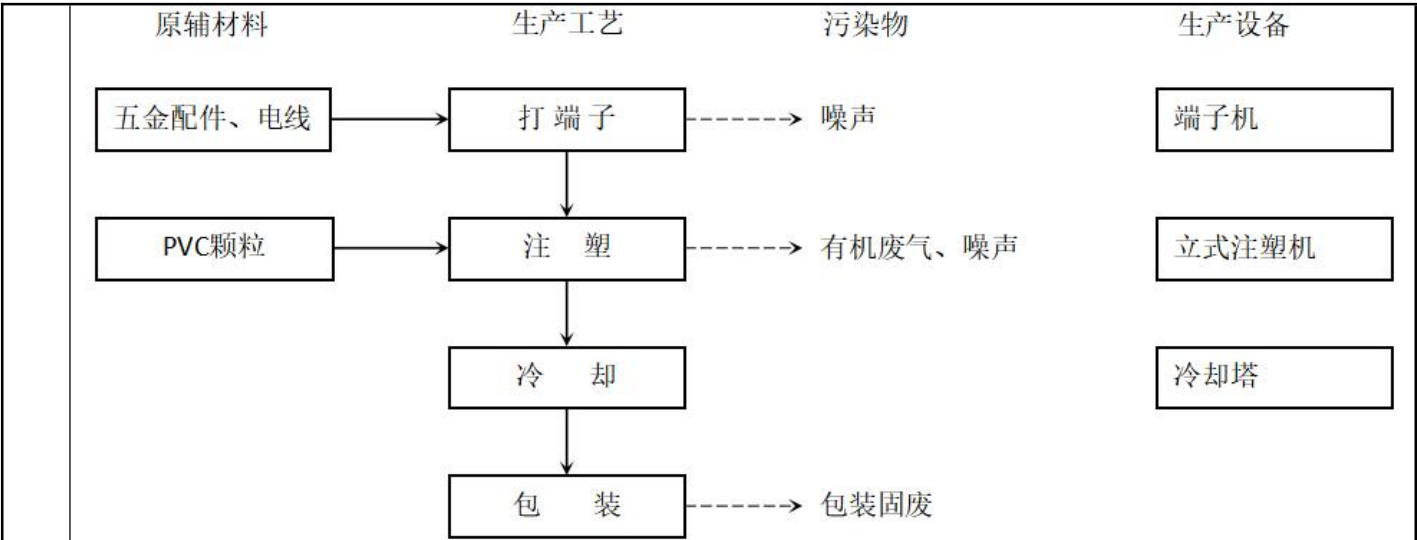
图 2-3 电源线生产工艺流程图
