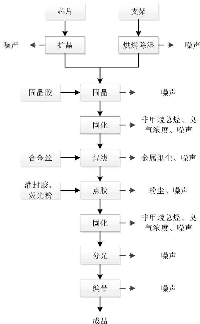
图 2. 生产工艺流程图
