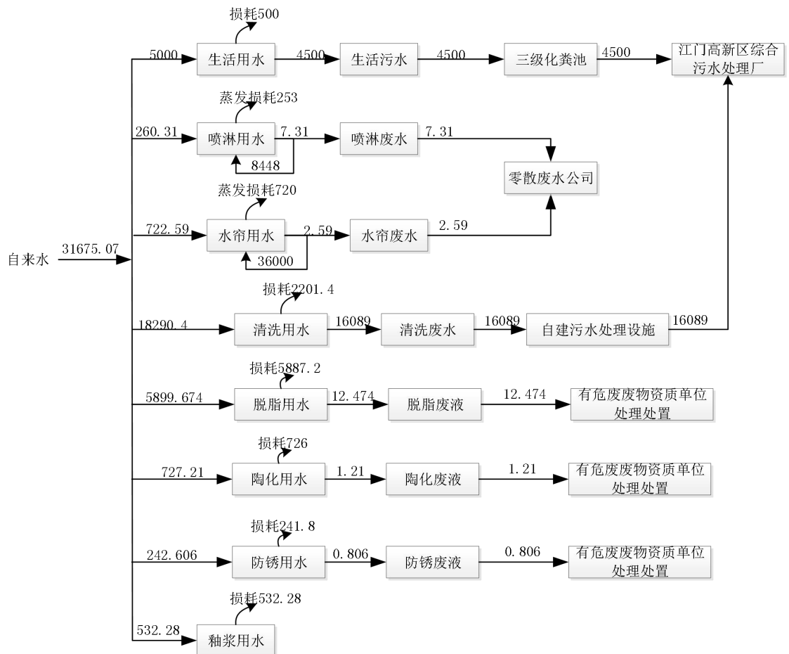
图 1 项目水平衡图
