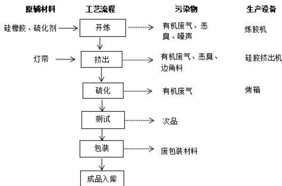
图 2-2 项目硅胶灯带生产工艺流程图
