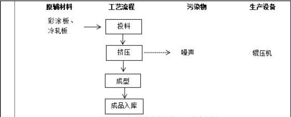
图 2-3 项目铁壳净化灯挤压工艺流程图
