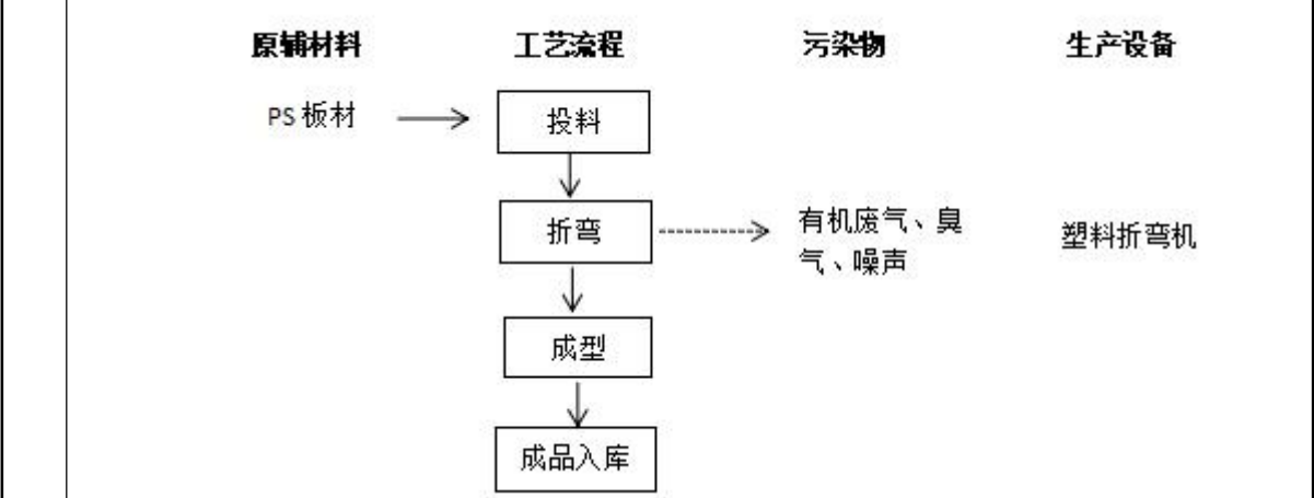
图 2-4 项目压花罩工艺流程图
