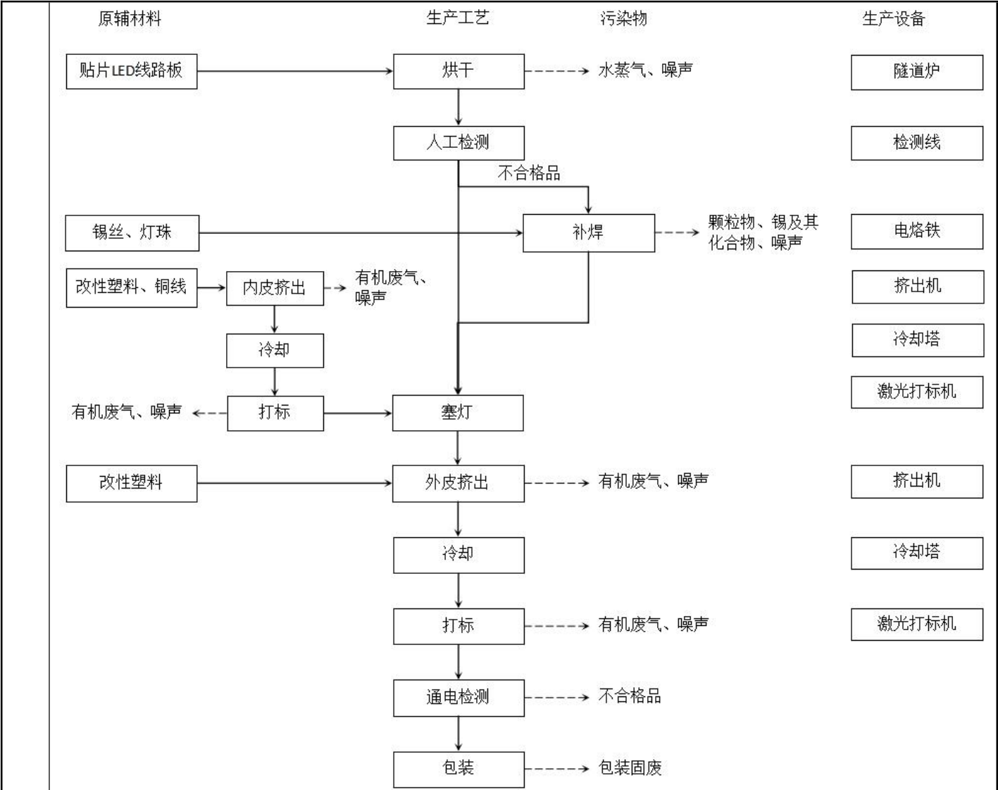
图2-3 LED灯带生产工艺流程图
