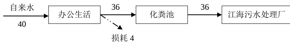
图 2-1 项目水平衡图 (单位: \text{m}^3/\text{a} )
