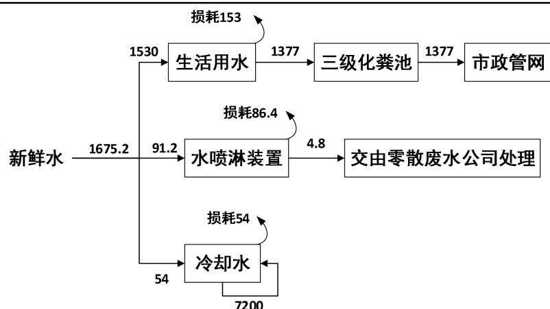
图 2-1 迁建项目水平衡图 单位: m³/a
