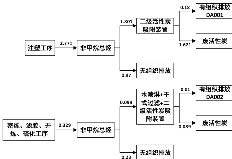
图 2-2 迁建项目 VOCs 平衡图 单位: t/a
