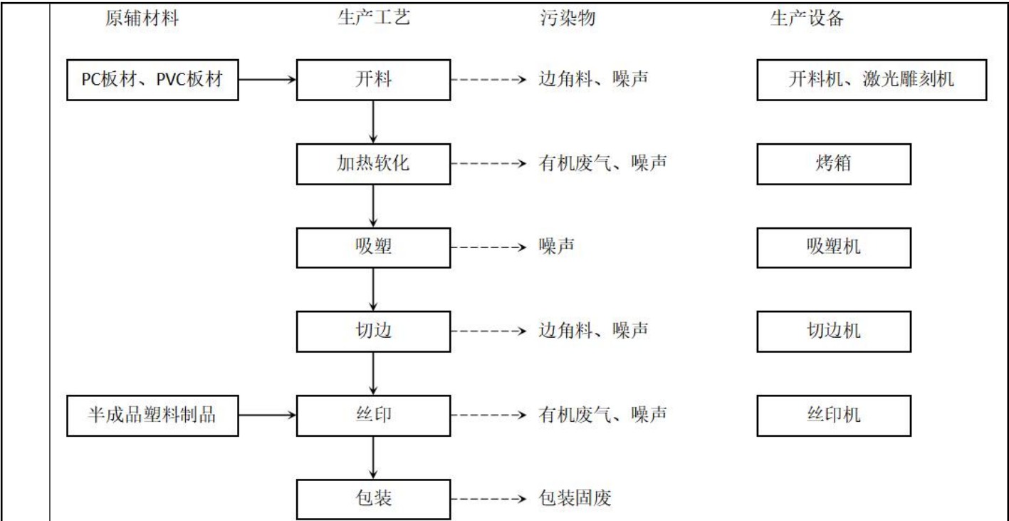
图2-2 塑料制品生产工艺流程图
