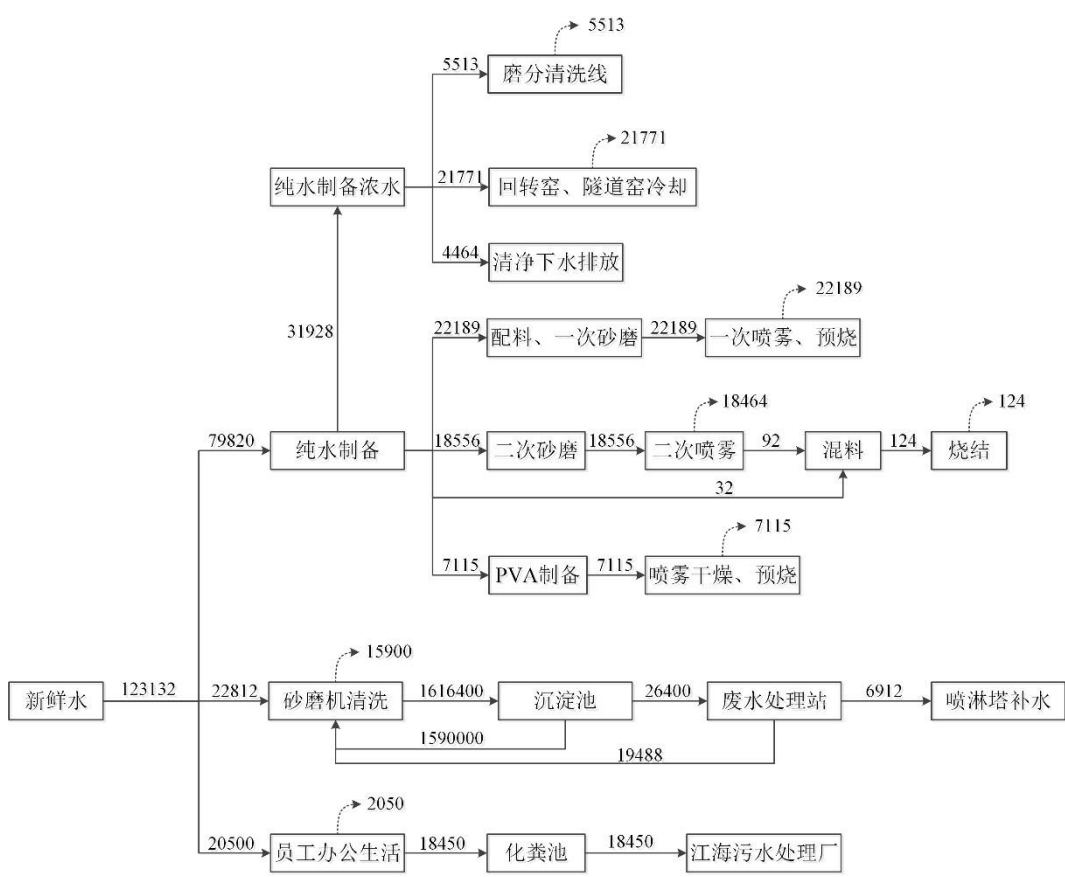
图 2-4 现有项目水平衡图
