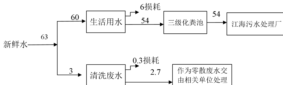
图 2-1 项目水平衡图 ( \text{m}^3/\text{a} )
