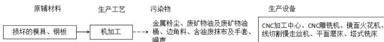
图 2-3 模具制造及维修生产工艺流程图
