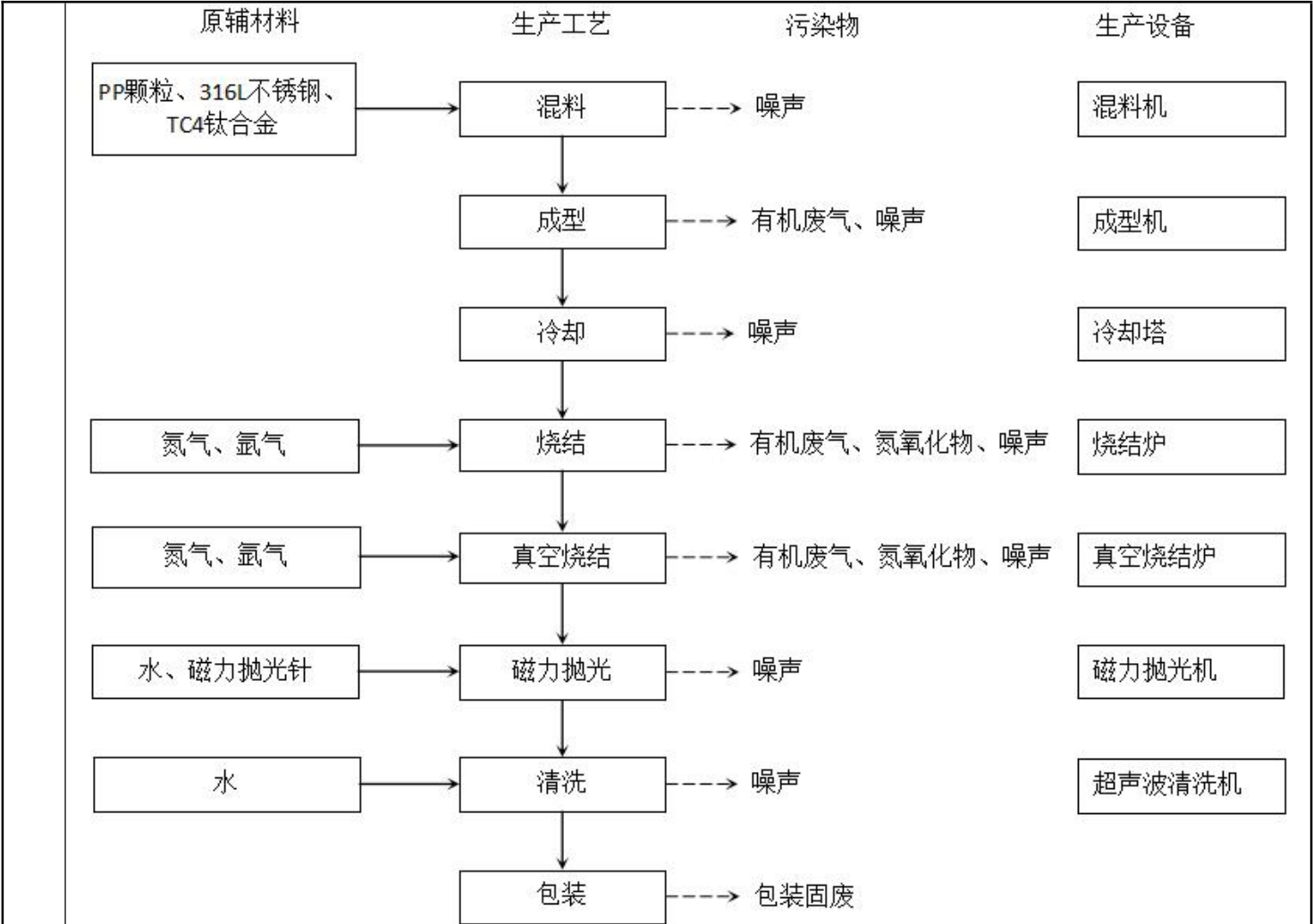
图2-2 生产工艺流程图
