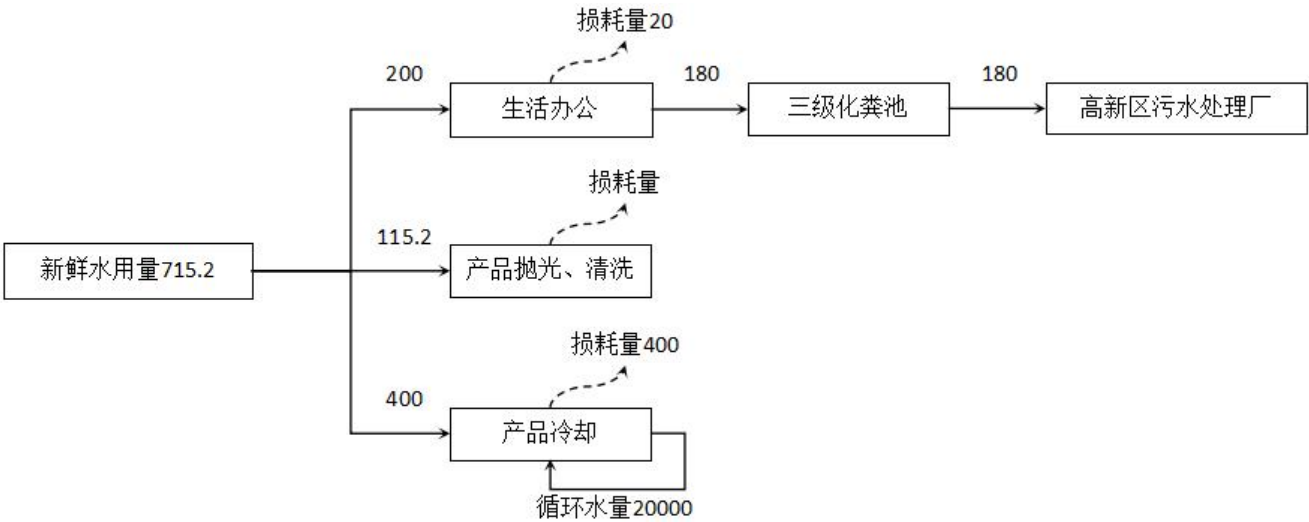
图 2-1 项目水平衡图 (t/a)
