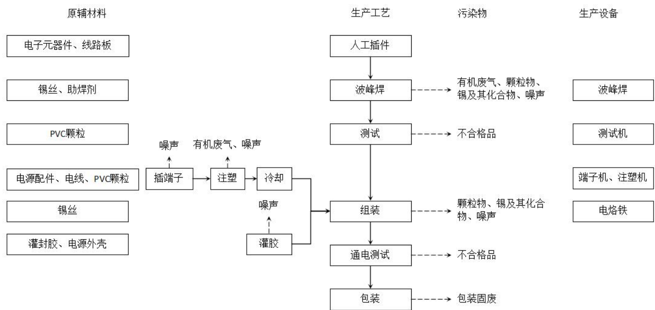
图 2-2 电源控制器生产工艺流程图
