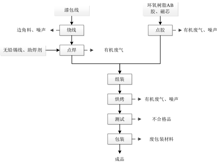
图1. 生产工艺流程图
