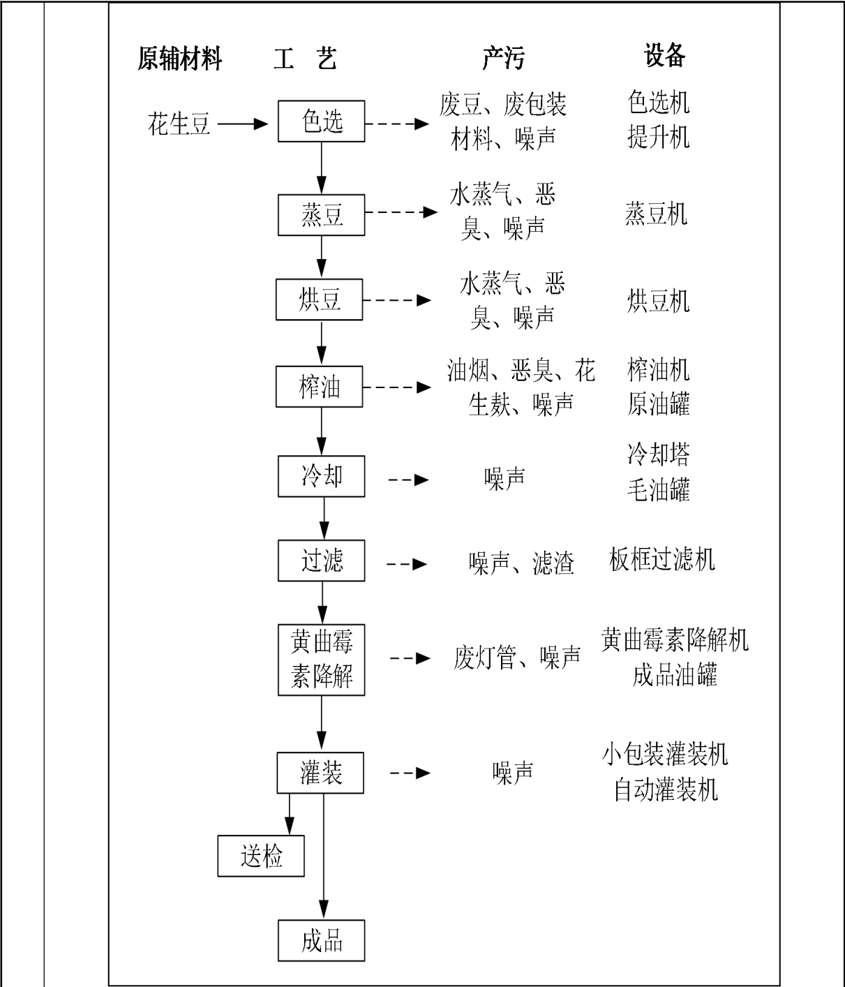
图 2-2 花生油生产工艺流程图
