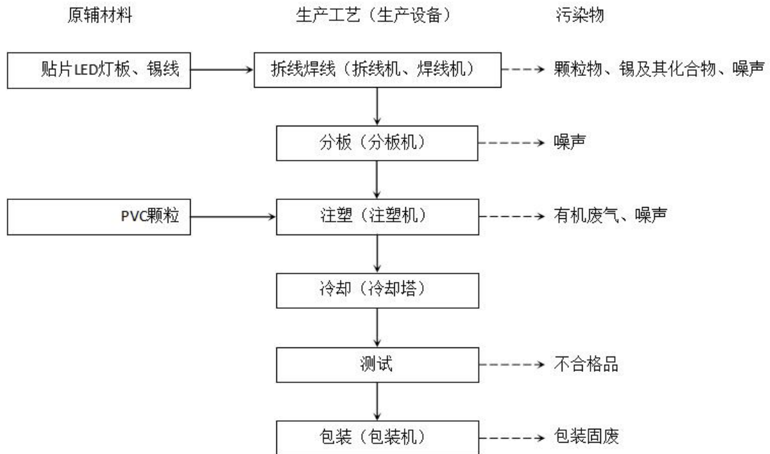
图2-2 LED模组生产工艺流程图
