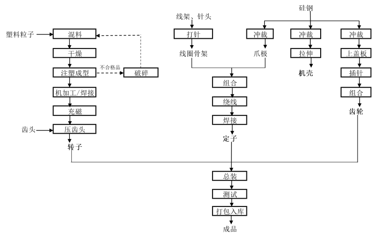
图 2-2 生产工艺流程图
